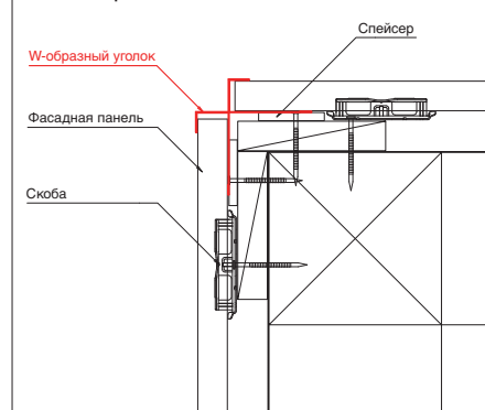
■ Схема крепления
